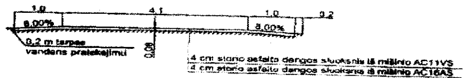
Pjūvis B-B
