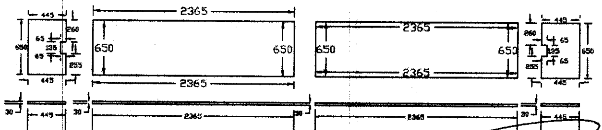
2 pav. Klevų g., esančio reprezentacinio ženklo, pjedestalo sutvarkymui skirtų granito plokščių matmenys
