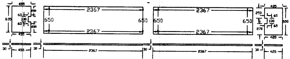
1 pav. V.Kudirkos g., esančio reprezentacinio ženklo, pjedestalo sutvarkymui skirtų granito plokščių matmenys
