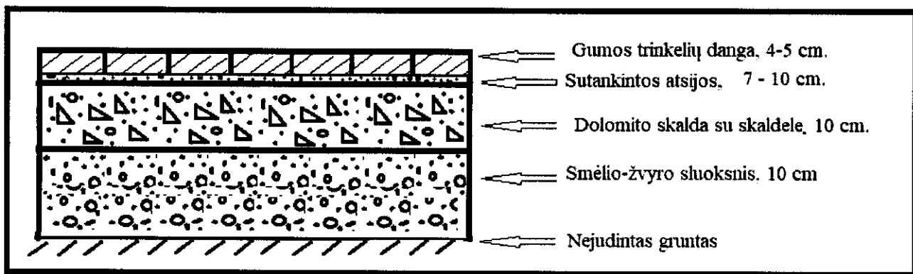
Dangų įrengimo schema
