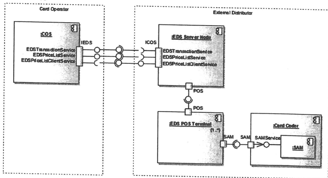
Pav. 1 Principinė e. bilių platintojumo sistemos veikimo schema
