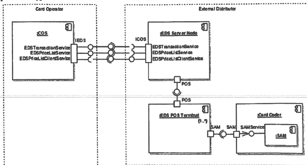
Pav. 1 Principinė e. bilietai platinimo sistemos veikimo schema
