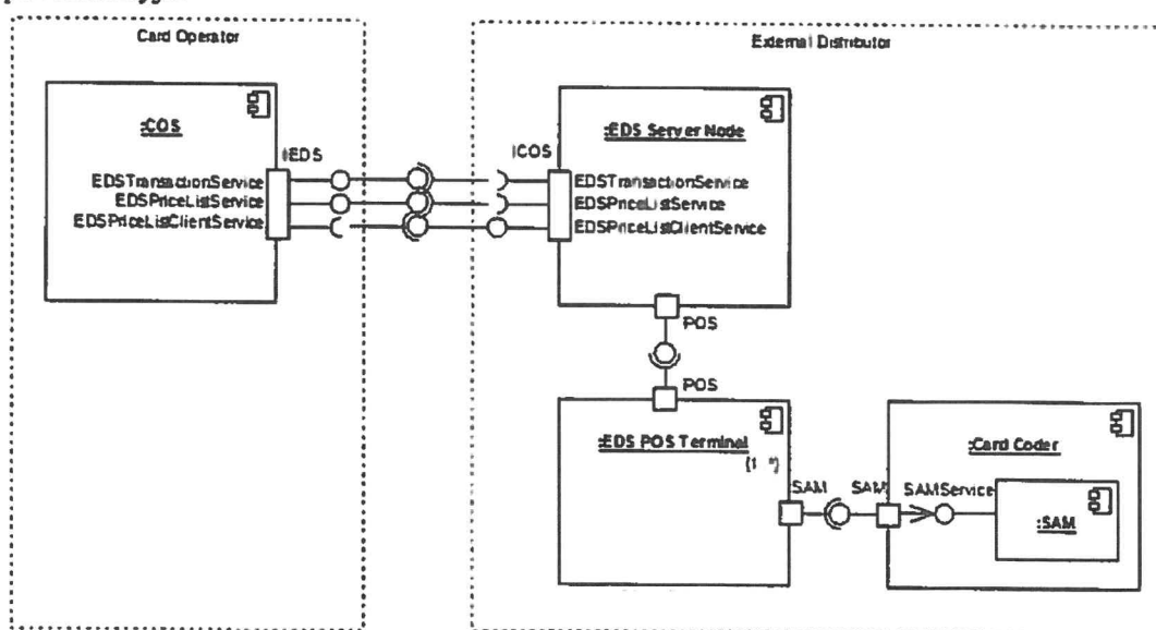
Pav. 1 Principinė e. bilieto platinimo sistemos veikimo schema
