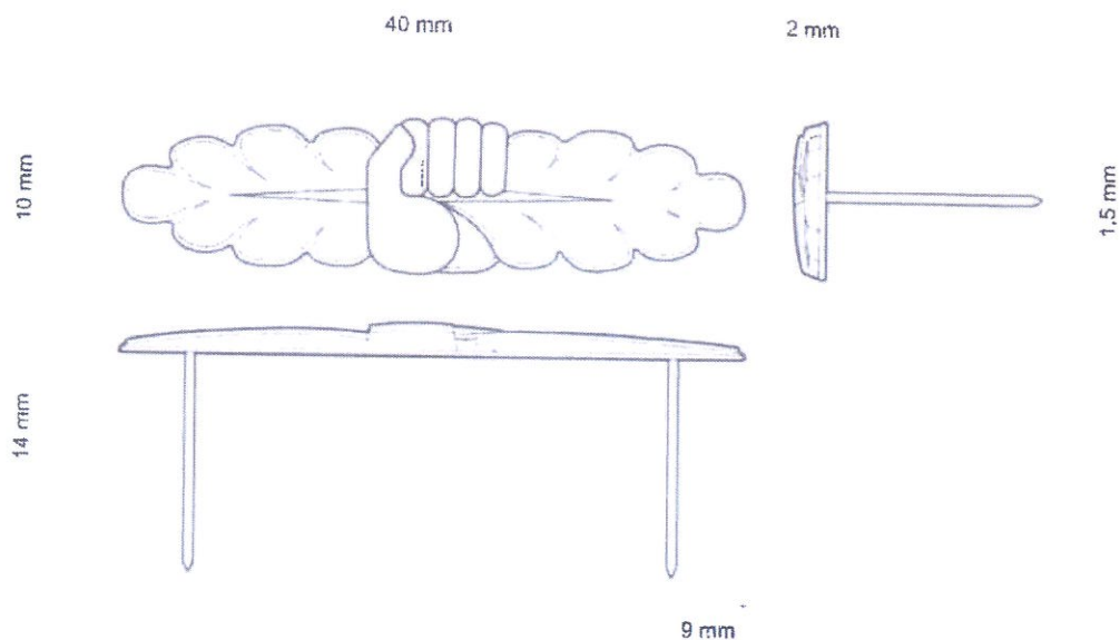
2 pav. Brėžinys M 2:1 ir aprašymas.
