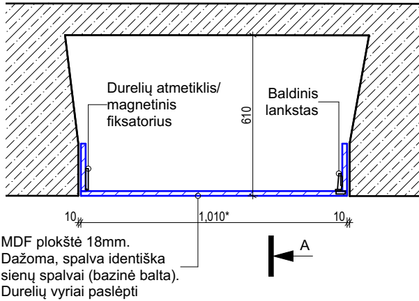
VAIZDAS PLANE
