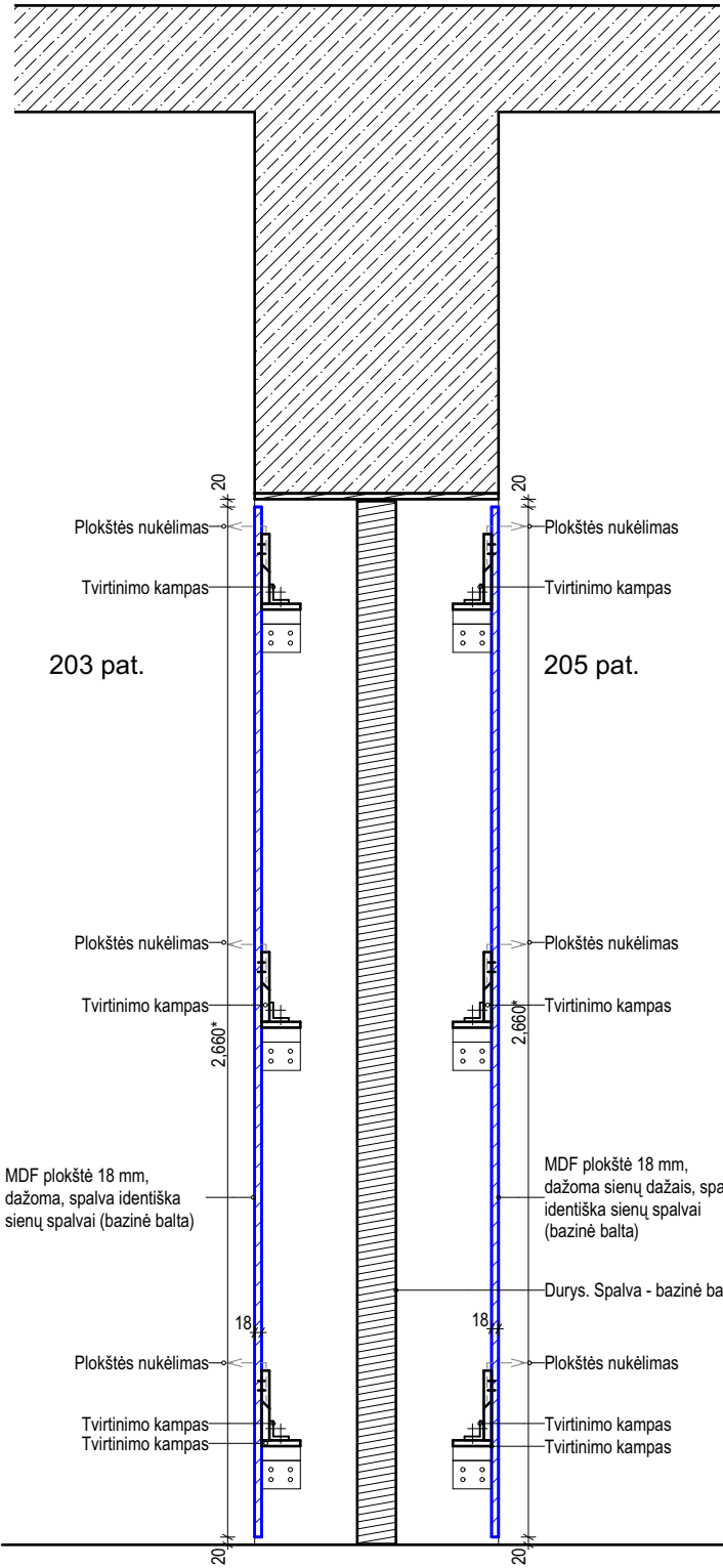
PJŪVIS A-A
