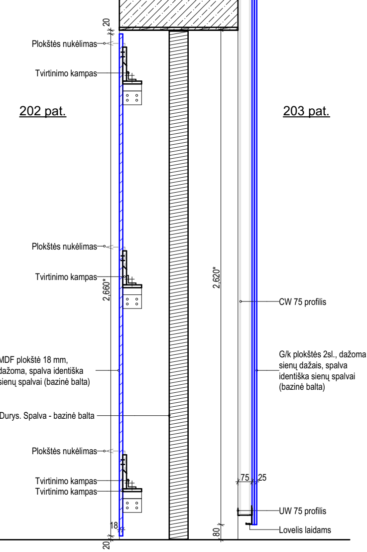
PJŪVIS A-A
