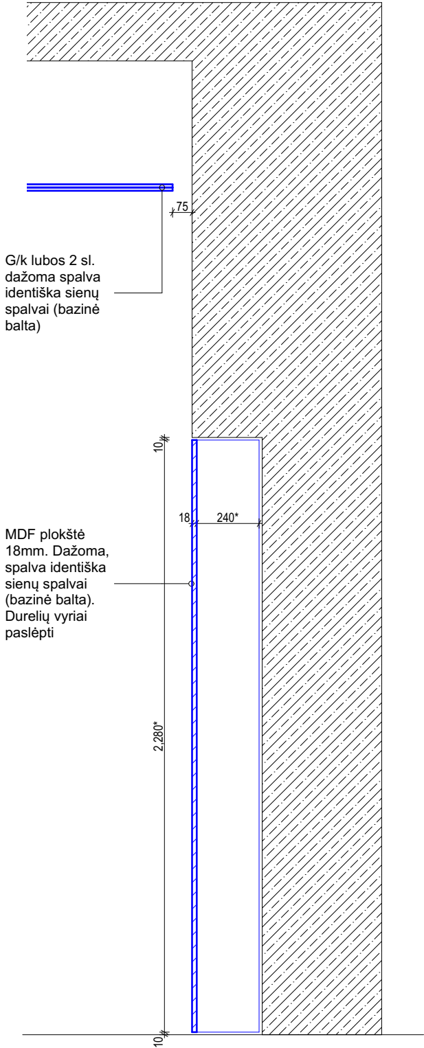
PJŪVIS A-A
