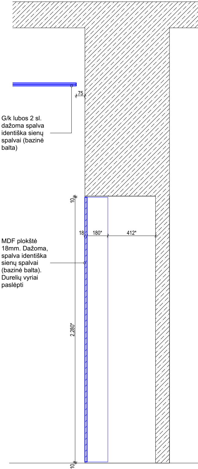
PJŪVIS A-A
