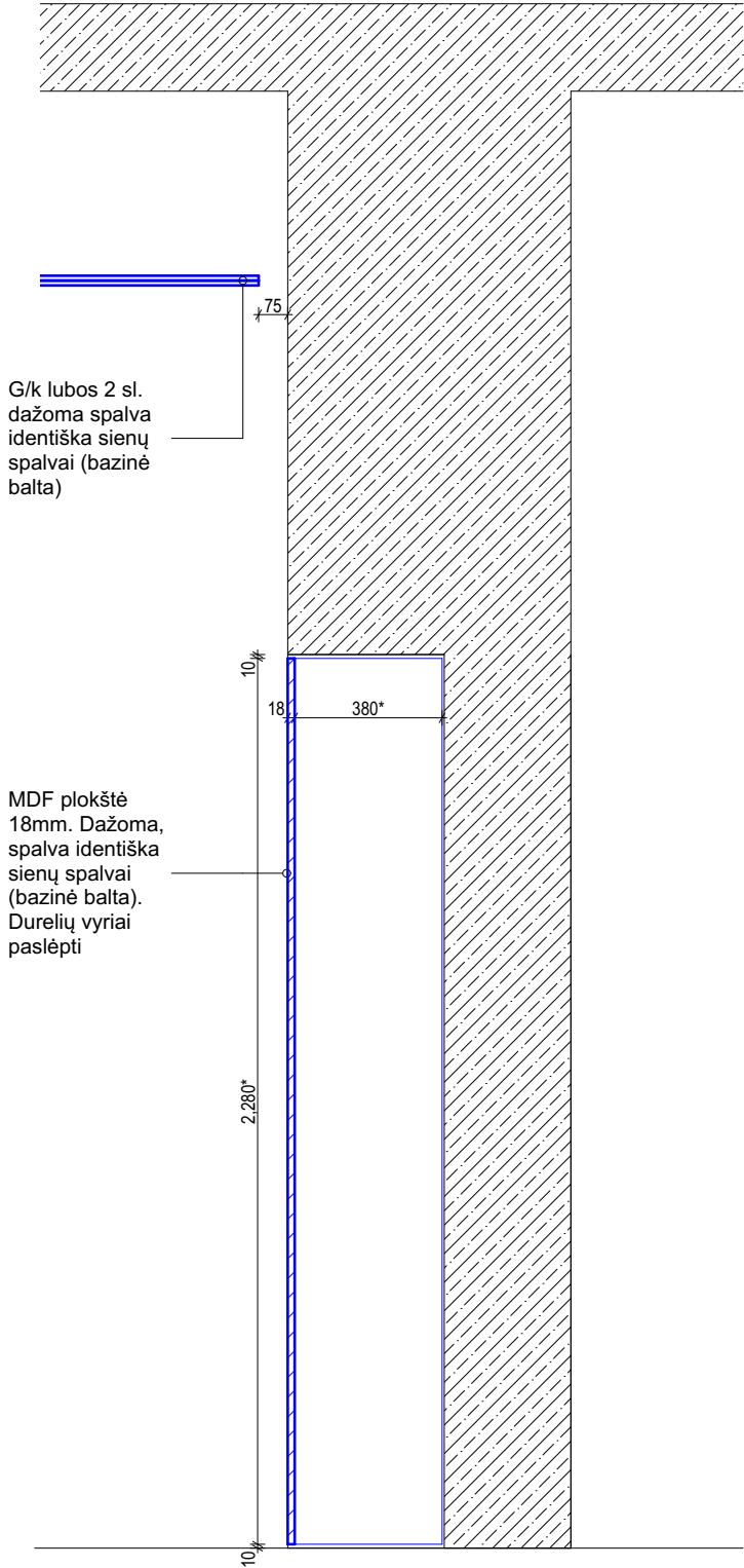
PJŪVIS A-A
