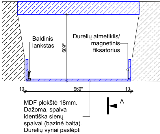
VAIZDAS PLANE
