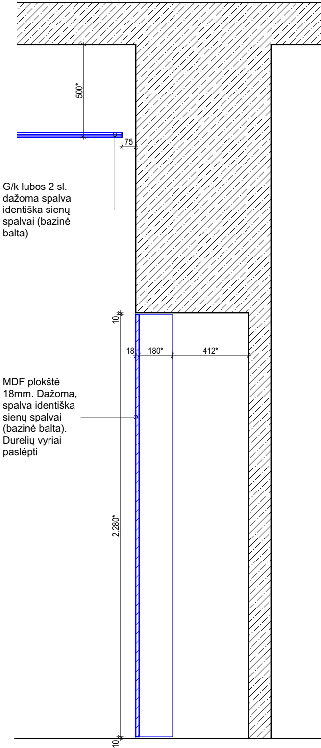
PJŪVIS A-A
