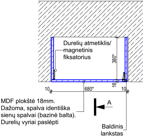
VAIZDAS PLANE
