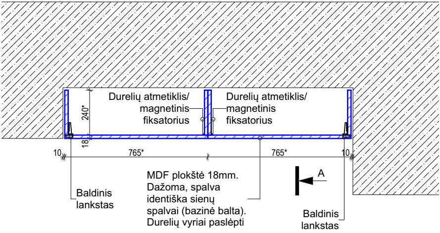
VAIZDAS PLANE
