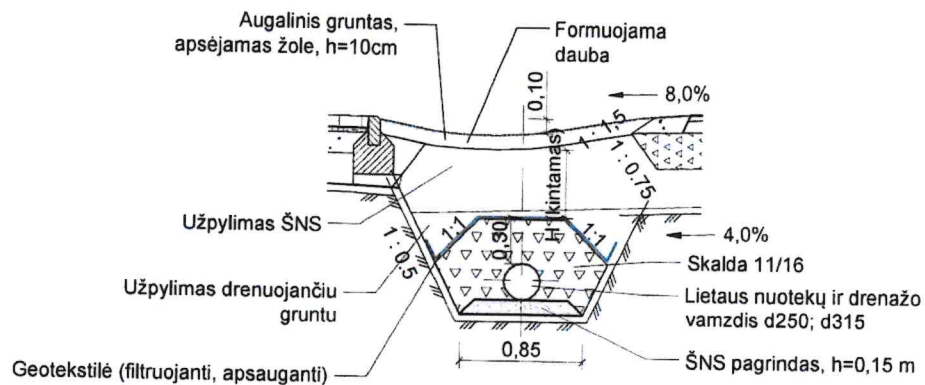
Lietaus nuotekų ir drenažo vamzdžių įrengimo schema M 1:50 (taikoma M. Valančiaus g. Pk 5+66 - Pk 6+84, dešinė)
