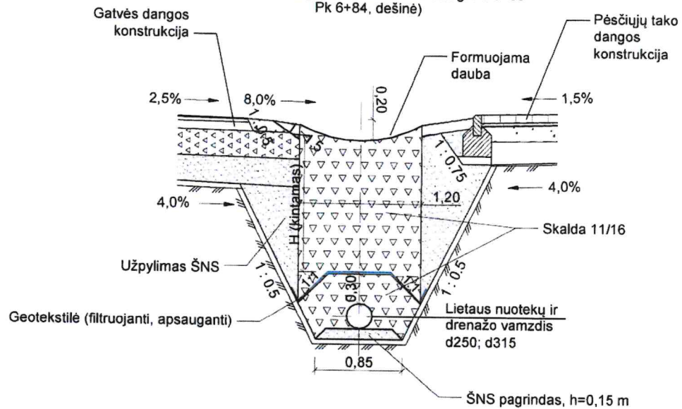
Lietaus nuotekų ir drenažo vamzdžių įrengimo schema M 1:50 (taikoma M. Valančiaus g. Pk 5+66 - Pk 6+84, dešinė)
