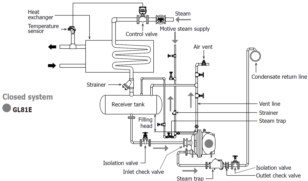
1 pav. Kondensato susigražinimo mazgo schema
