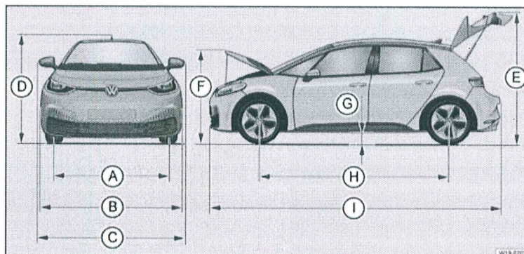
pav. 1 Matmenys.
