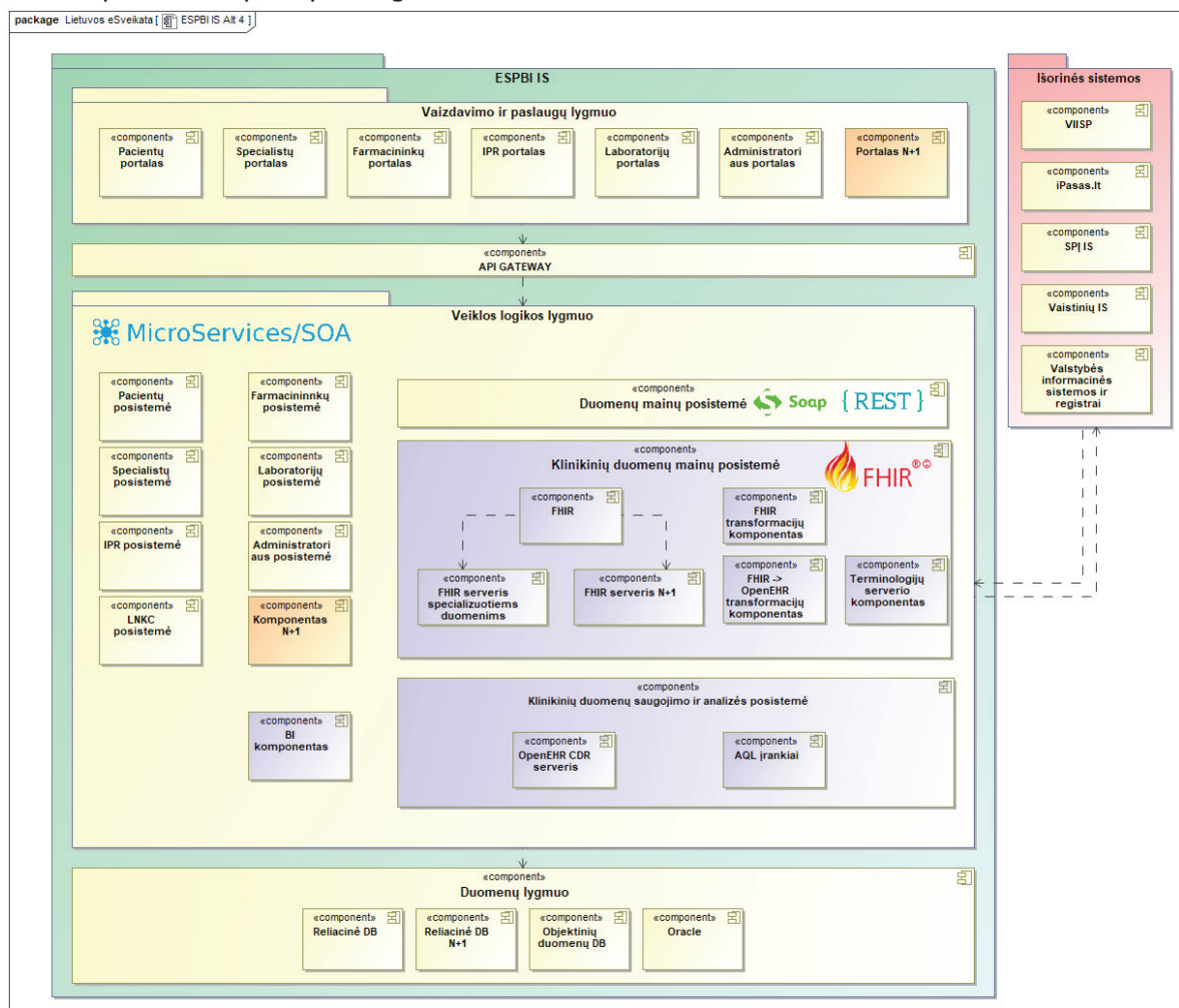
1. Pav. ESPBI IS loginės architektūros schema
