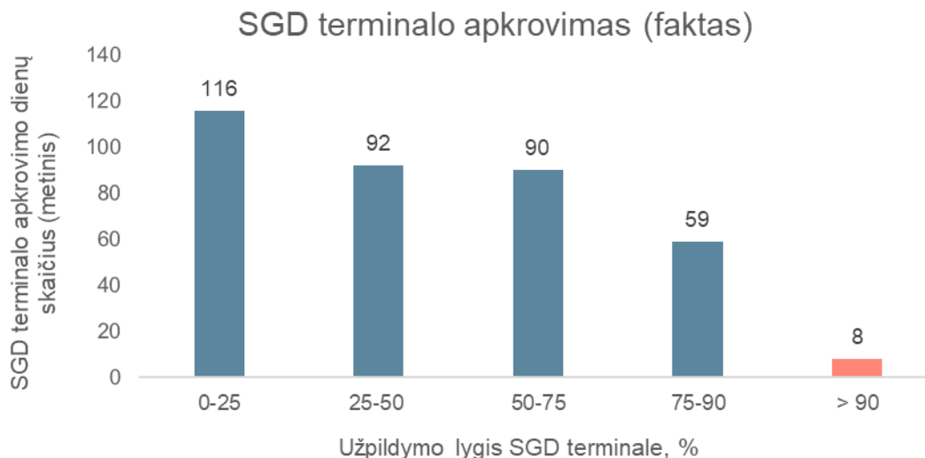
Paveikslas 5 "Independence" SGD terminalo apkrovimas 2024 m. sausio – rugpjūtis mėnesiais, įtraukiant 2024 m. rugpjūtis – gruodžio prognozę
