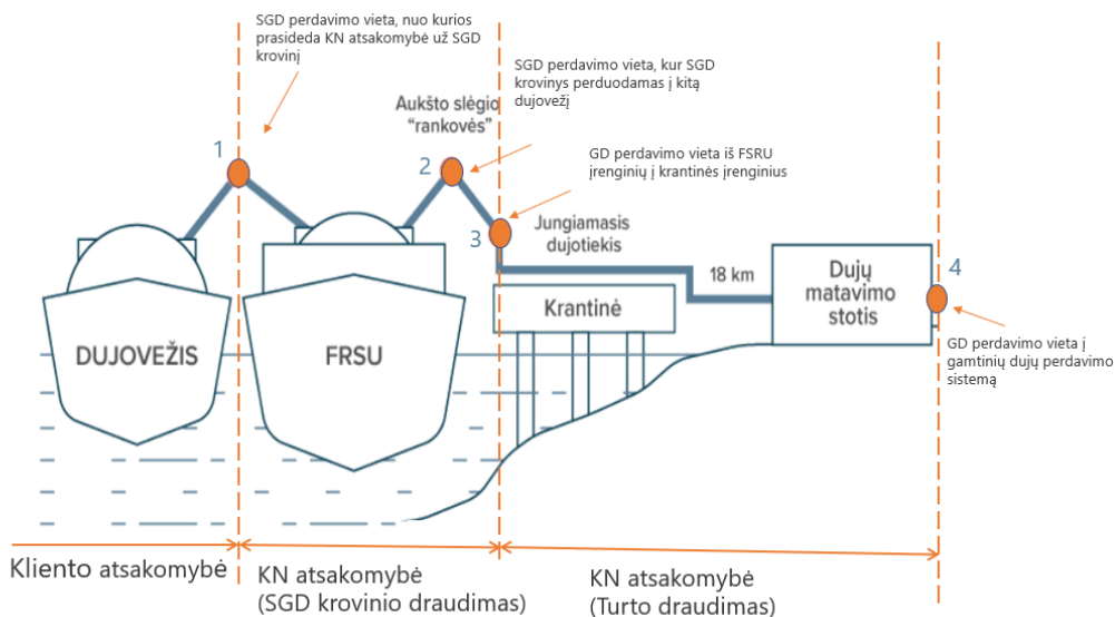
Paveikslas 1 SGD ir GD judėjimo schema SGD terminale
