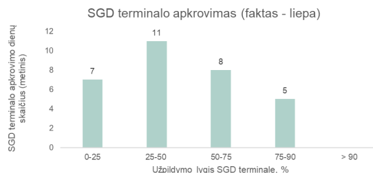
Paveikslas 7 "Independence" SGD terminalo apkrovimas liepos mėnesį (faktas)
