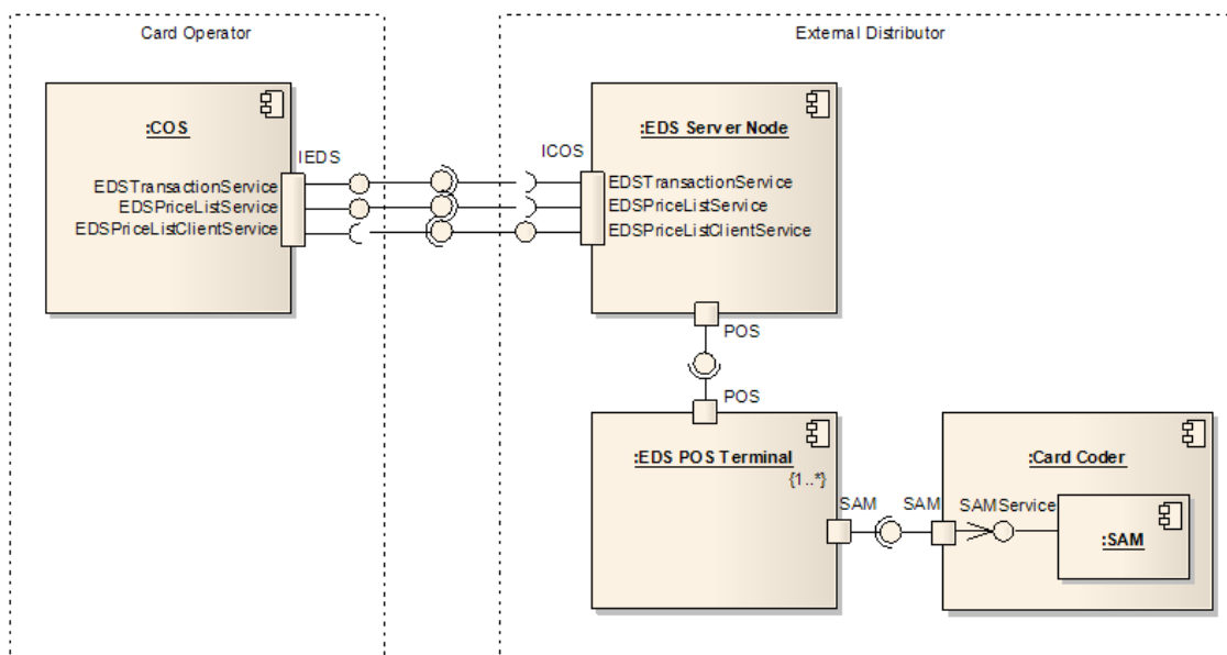
Pav. 1 Principinė e. bilietauto platintojų sistemos veikimo schema
