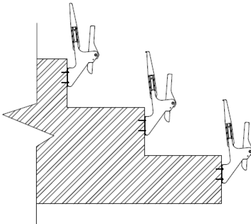
1 paveikslas. Kėdučių prie konstrukcijos tvirtinamo schema
