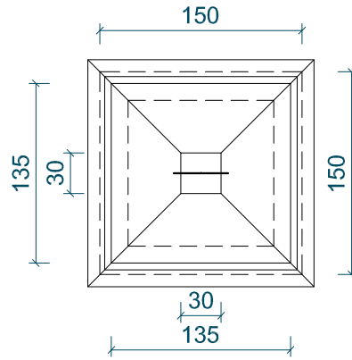
D-D
