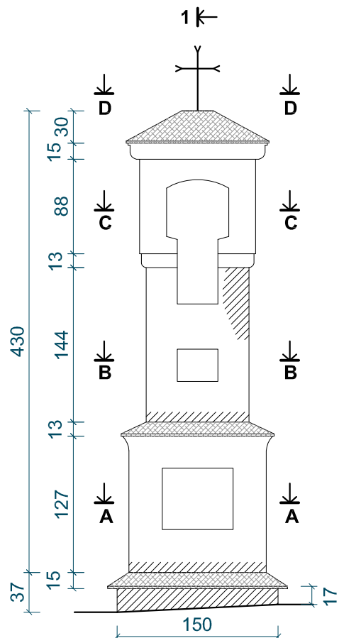
Š FASADAS M 1:50
