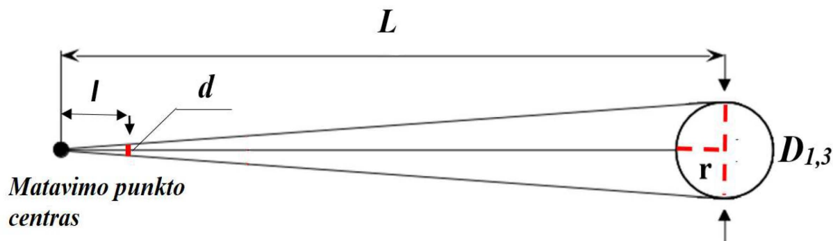
2 pav. V. Biterlichio pasiūlyto būdo medyno skerspločių sumai nustatyti schema
