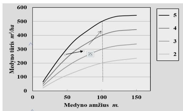
5 pav. Medyno tūrio indekso nustatymo normatyvų fragmentas. Skaičiai – medyno tūrio indeksas. Rodyklės vaizduoja, kad medynas ilgainiui gali keisti tūrio indeksą.
