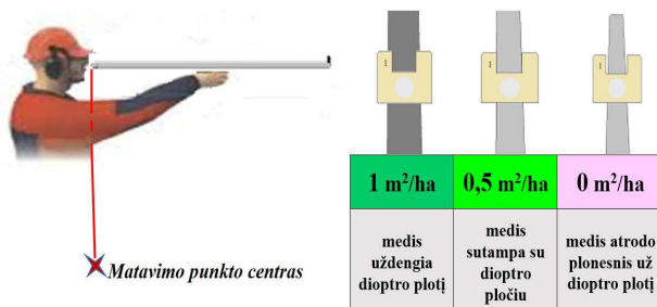
3 pav. Medyno skerspločių sumos matavimas su V. Biterlichio prietaisu
