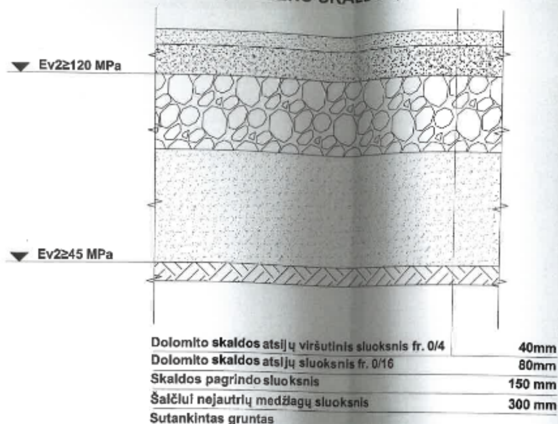
DETALĖ - 8, AKMENS SKALDOS, ATSIJŲ TAKAI
