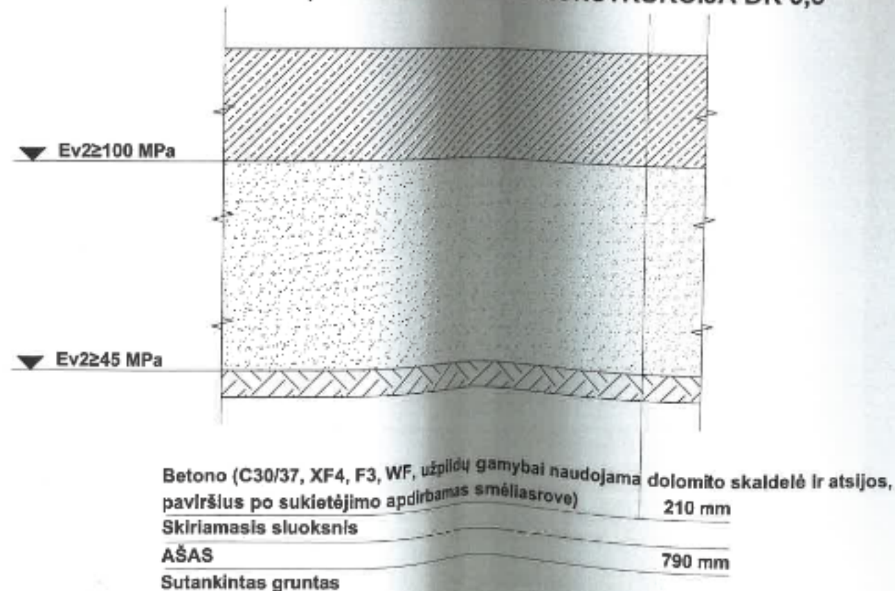
DETALĖ - 10, BETONO DANGOS KONSTRUKCIJA DK 0,3
