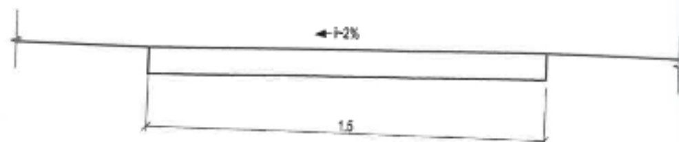
1.5 M. PLOČIO TAKO SALOJE SKERSINIS PJŪVIS M 1:20
