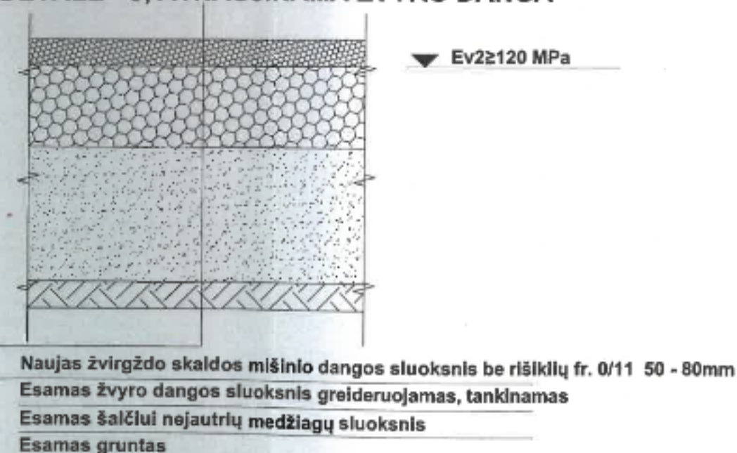
DETALĖ - 9, ATNAUJINAMA ŽVYRO DANGA
