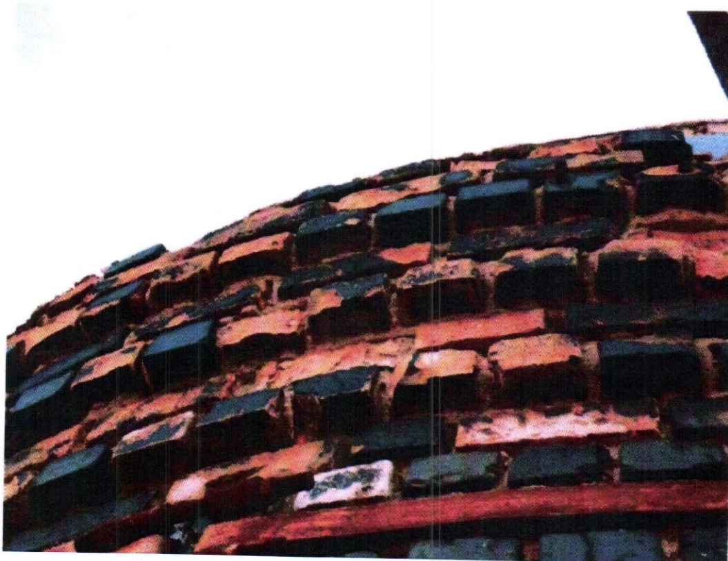
Viršūnės mūras įtrūkės 2 vnt. vertikaliais įtrūkiais 1,0-1,7 m ilgio, 2-10 mm pločio.
