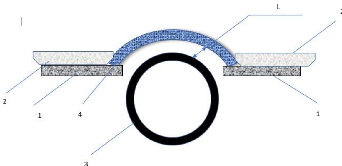
Pav. Nr.1 Gelžbetoninio kevalo įrengimo principinė schema.
