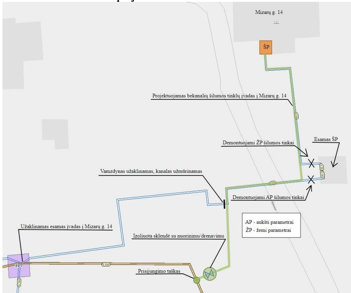
1 schema „Šilumos tiekimo tinklų nuo ŠK 8V-1 iki pastato Mizarų g. 14, Druskininkuose, rekonstravimo projektas“
