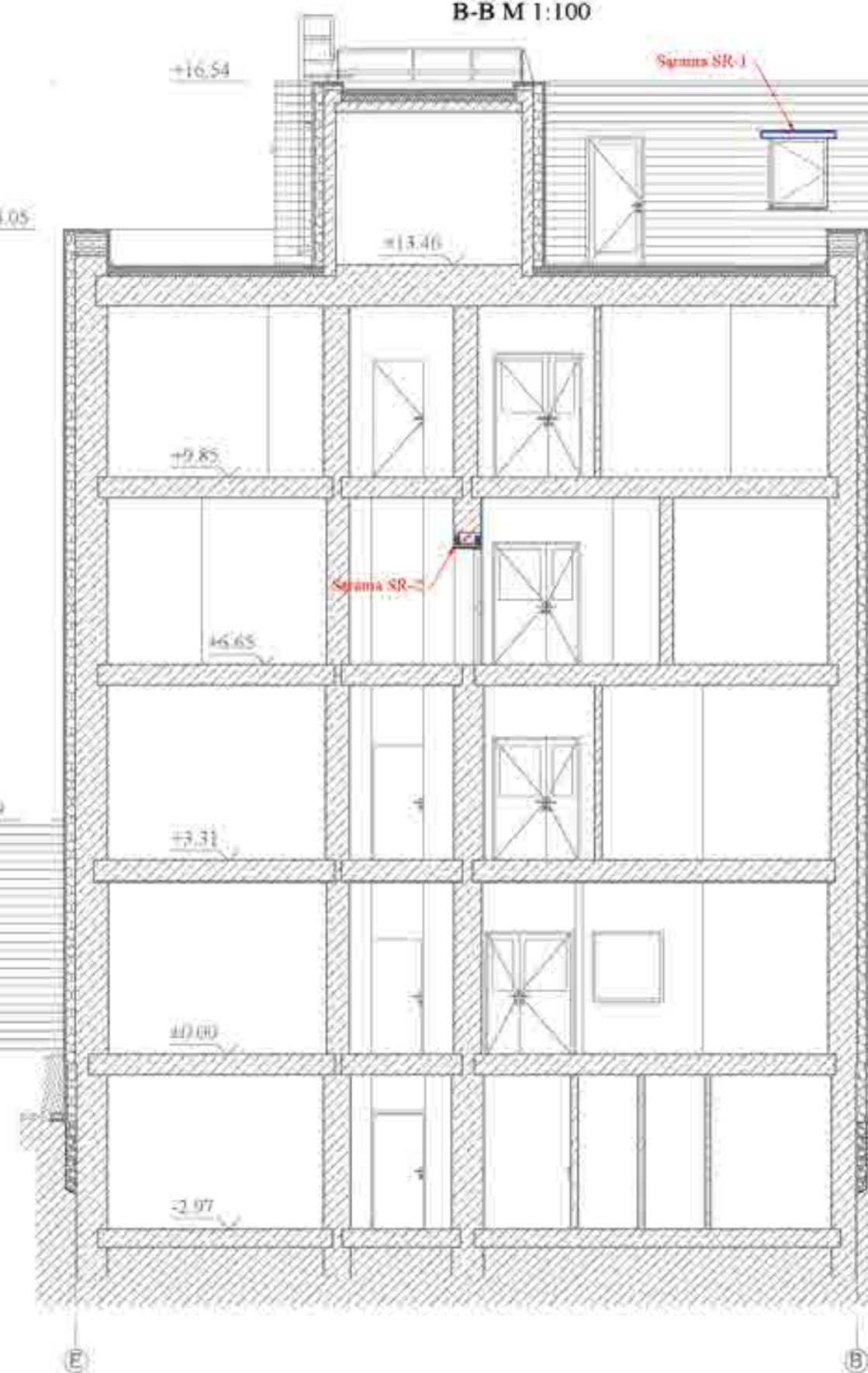
B-B M 1:100
