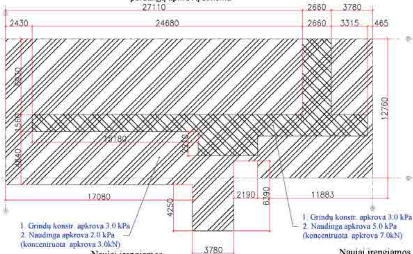
Naujai įrengiamos sėamos rūsyje apkrovų schema
