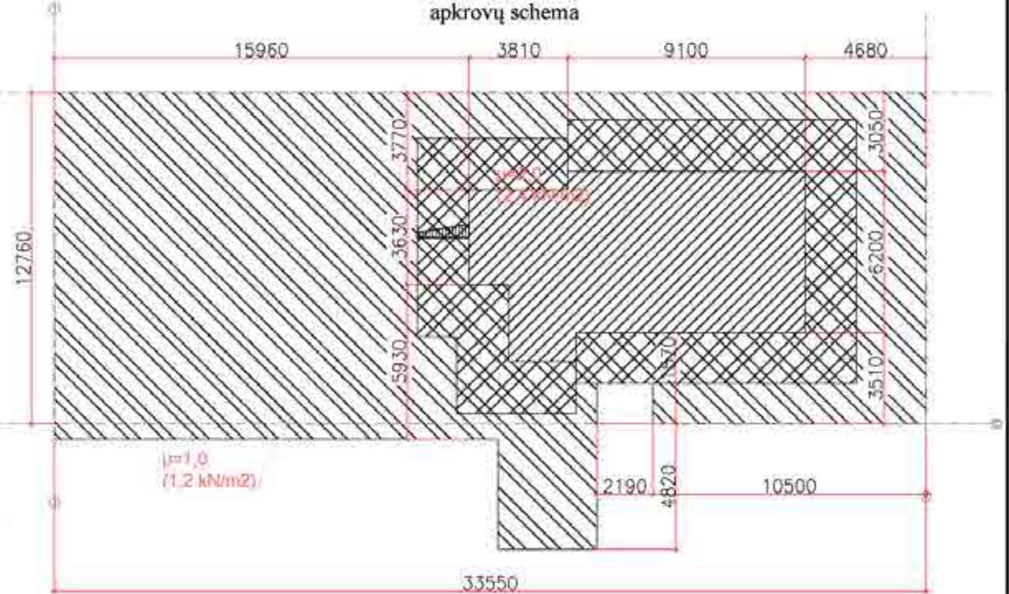
1. Grindų konstr. apkrova 2.5 kPa 2. Naudinga apkrova 2.0 kPa (koncentruota apkrova 3.0 kN)
