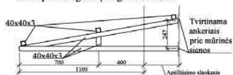
Principinė stogelio įrengimo schema
