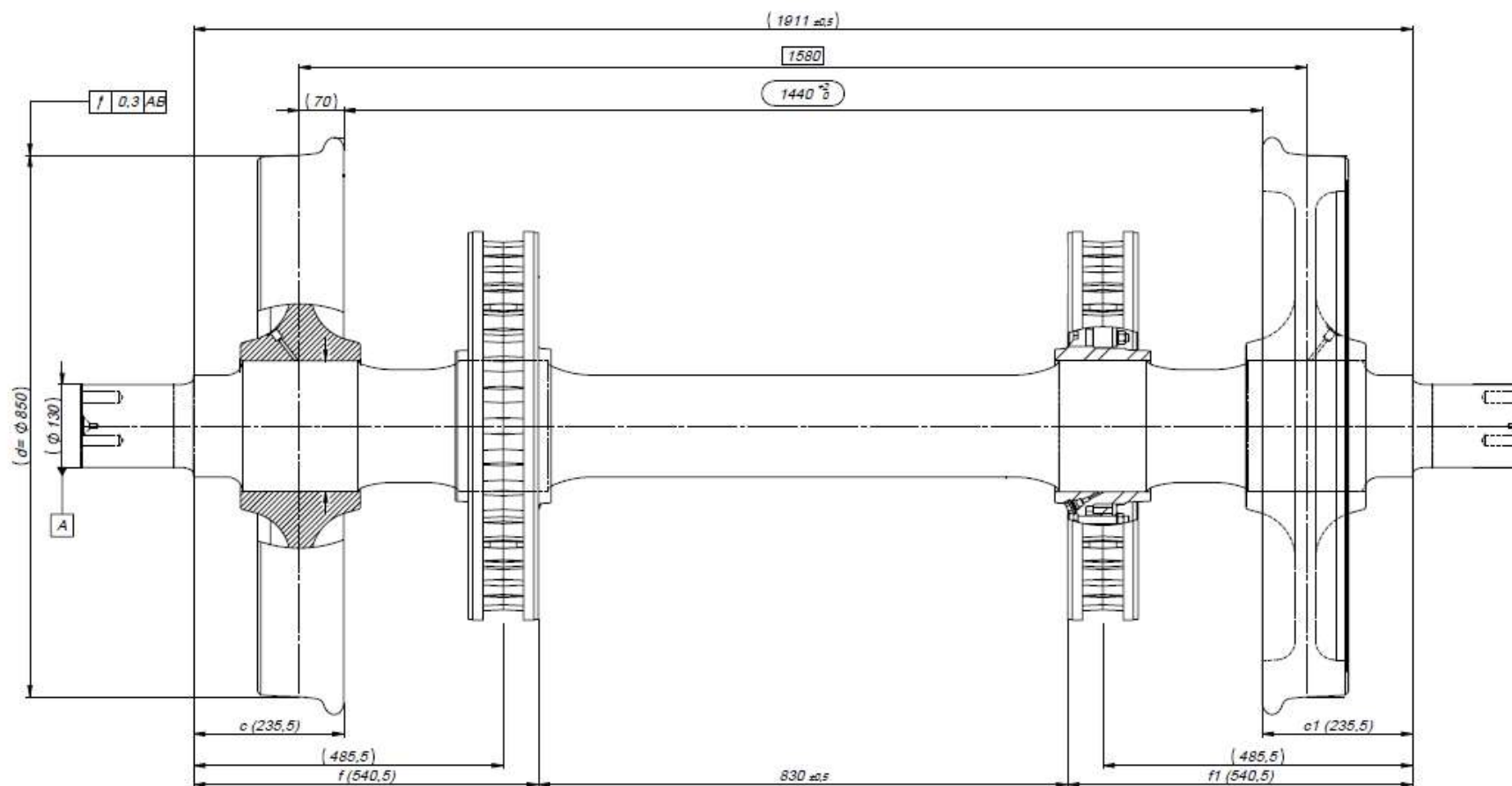
Dyzelinių traukinių PESA 630MiL palaikančiųjų aširačių brėžinys Nr. 11ASb 090101-1-00 (P0)
