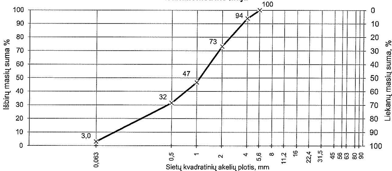
Granulimetrinė linija
