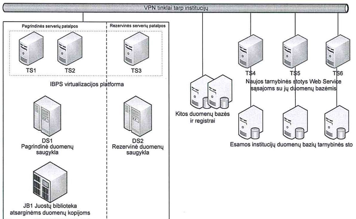
IBPS fizinė architektūra.
