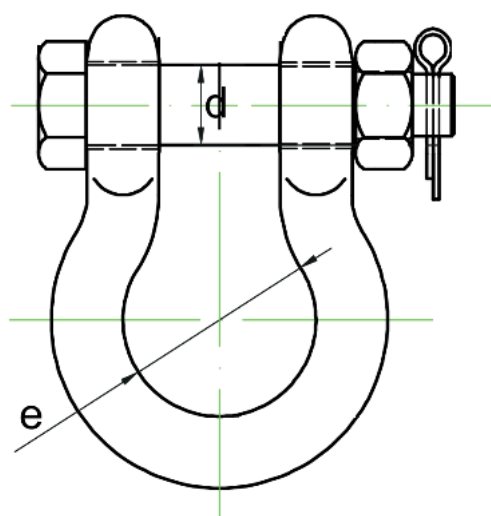
2 pav. Jungtis
