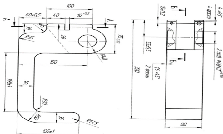
1 pav. Keturkampio vamzdžio griebtuvas
