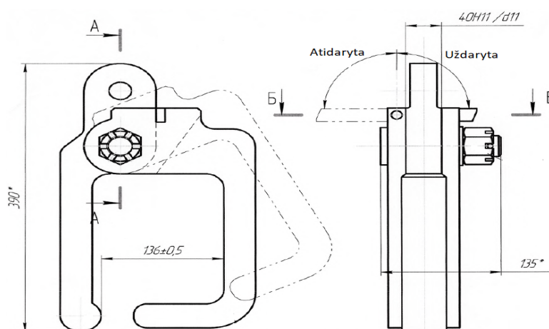
2 pav. Keturkampio vamzdžio griebtuvas
