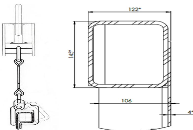
3 pav. Keturkampis vamzdis
