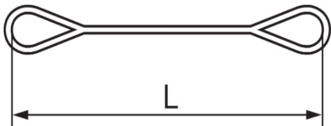
1 pav. Sintetinio pluošto juostinis stropas su kilpa abiejuose galuose
