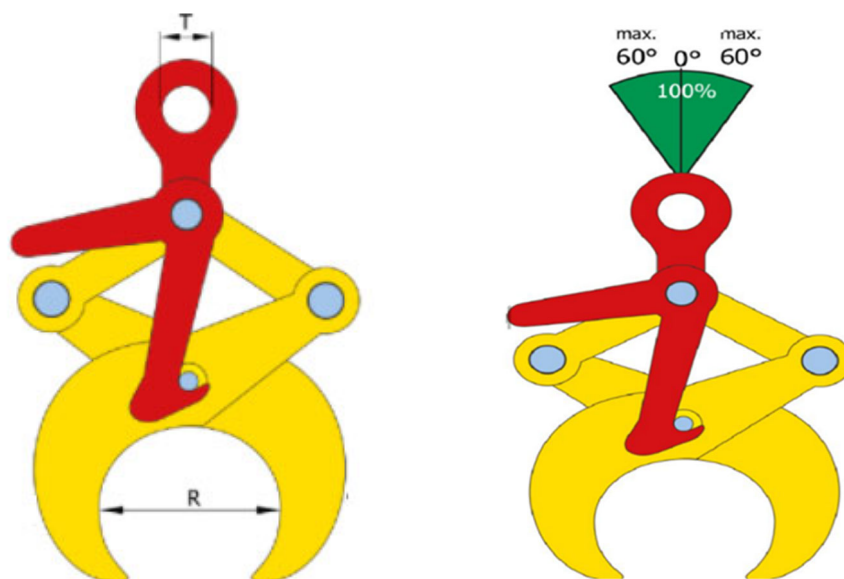
1 pav. Žirklinis griebtuvas
