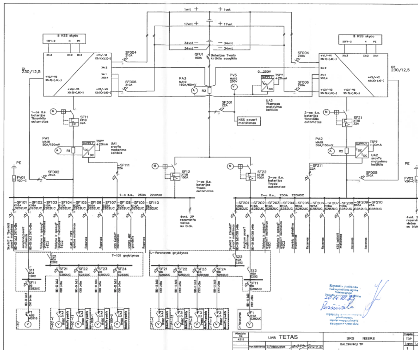
Šalčininkų TP nuolatinės srovės sąvųjų reikmių schema
