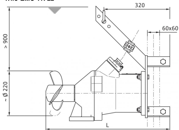
Brėžinys Wilo-EMU TR 22
