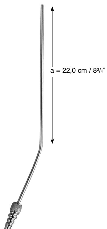
YASARGIL 017-476-015 Ø 1,5 mm 017-476-020 Ø 2,0 mm 017-476-025 Ø 2,5 mm 017-476-035 Ø 3,5 mm
