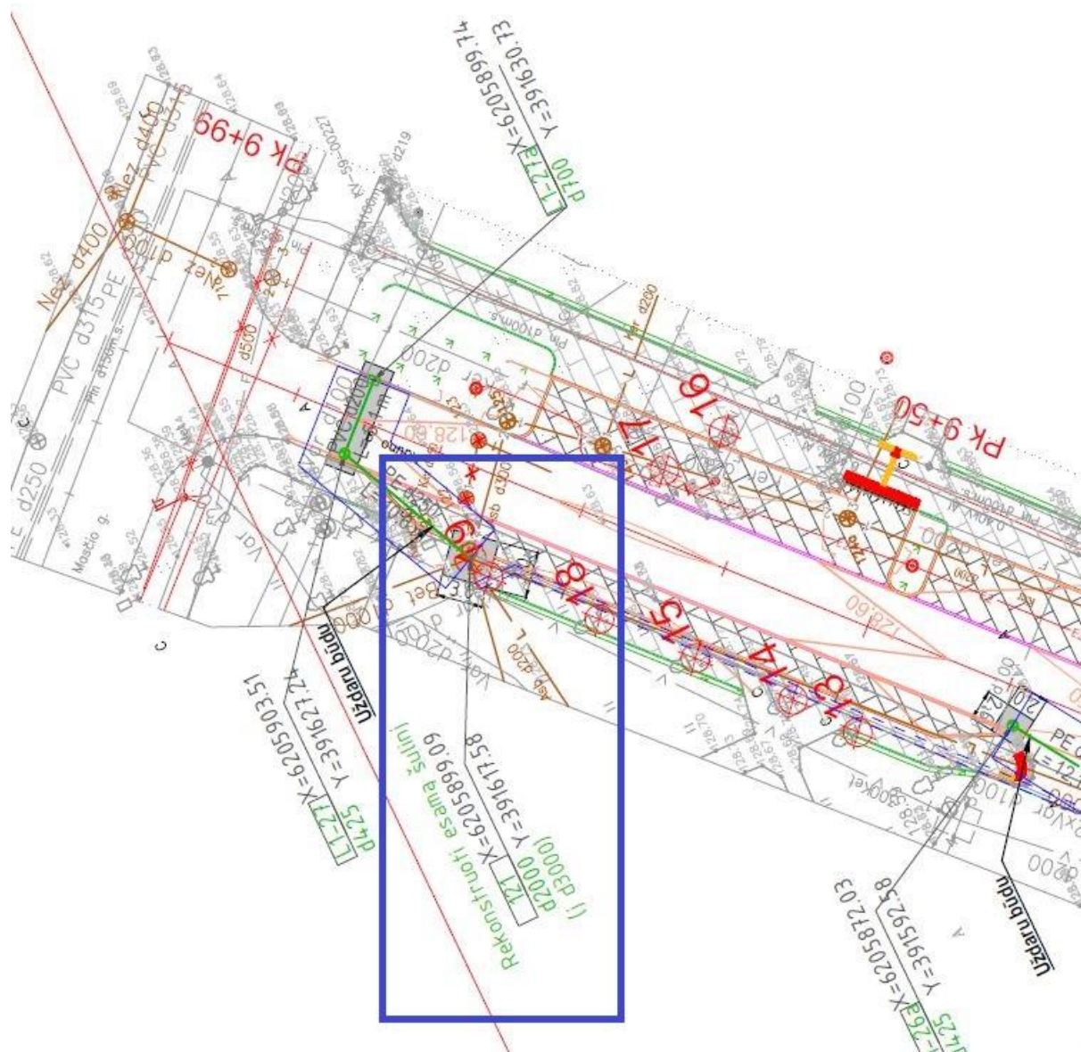
2 pav. Esamo d2000 g/b šulinio Nr. 121 vieta
