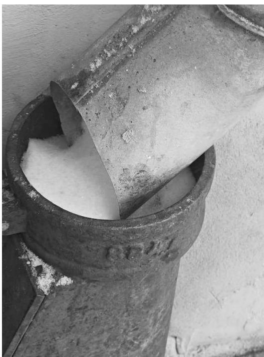
8 pav. 3.2.p. pastebėti lietaus ir buitinių nuotekų tinklų defektai.
