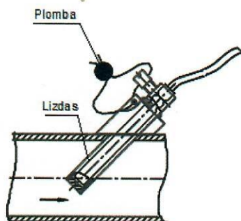
10 pav. PL tipo temperatūros zondų plombavimas
