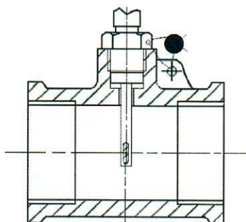
10 pav. PL tipo temperatūros zondų plombavimas
