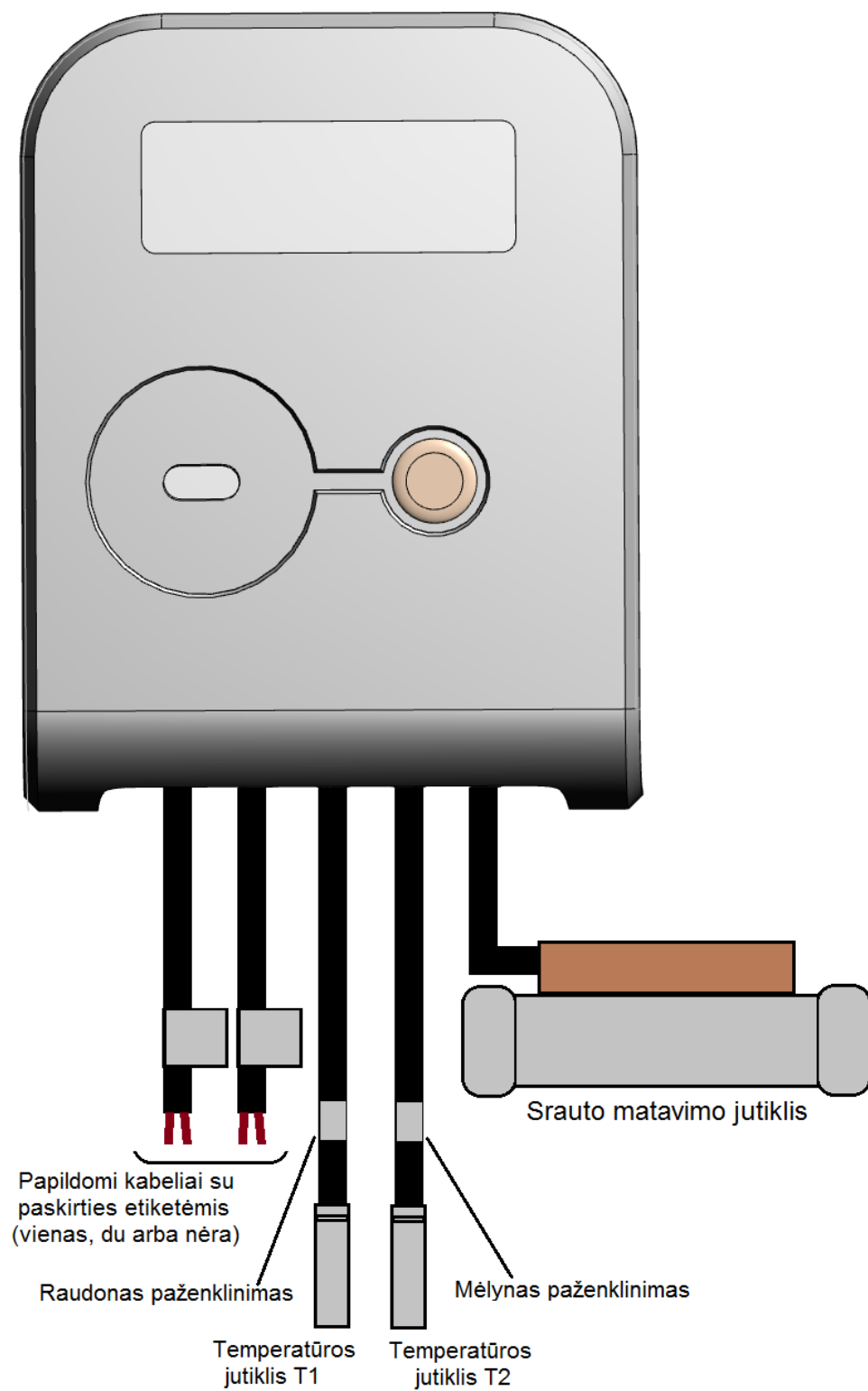
A1 pav. Skaitiklio prijungimo schema. Konstrukcinis variantas su nekeičiamai prijungtais temperatūros jutikliais.
