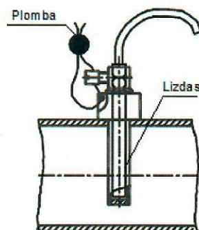
10 pav. PL tipo temperatūros zondų plombavimas
