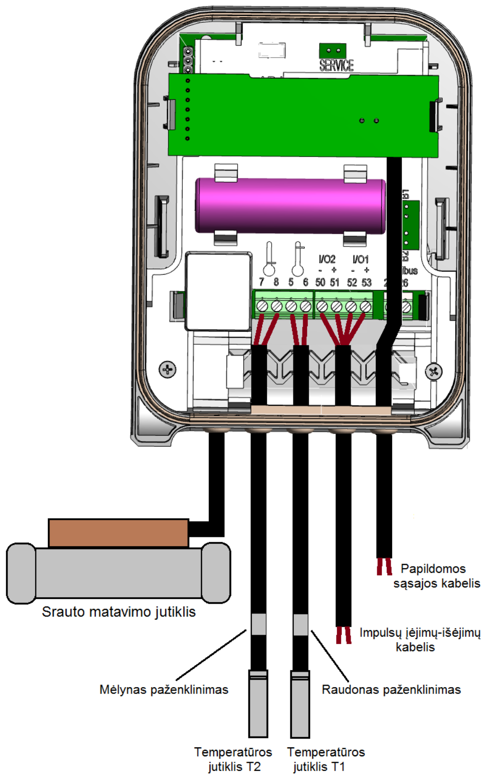
A3 pav. Skaitiklio prijungimo schema. Konstrukcinis variantas su keičiamais temperatūros jutikliais ir papildoma sąsaja (sąsajos modulis montuojamas prieinama atkėlus modulį).
