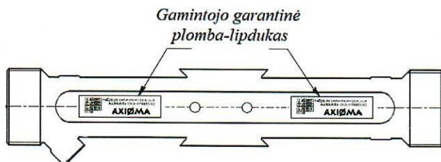
c) srauto jutiklio q_p = 3,5 \text{ m}^3/\text{h} plombavimas (apvalaus skerspjuvio matavimo kanalas)
