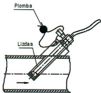
9 pav. PL tipo temperatūros zondų plombavimas
