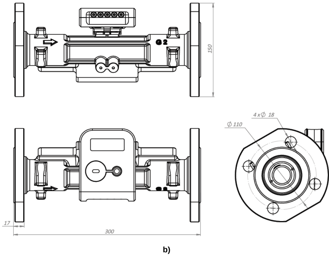
B2.6 pav. Srauto jutiklis q_p = 10,0 \text{ m}^3/\text{h} ; L=300 \text{ mm} a) prijungimo tipas: sriegis G2"; b) prijungimo tipas: jungės DN40
