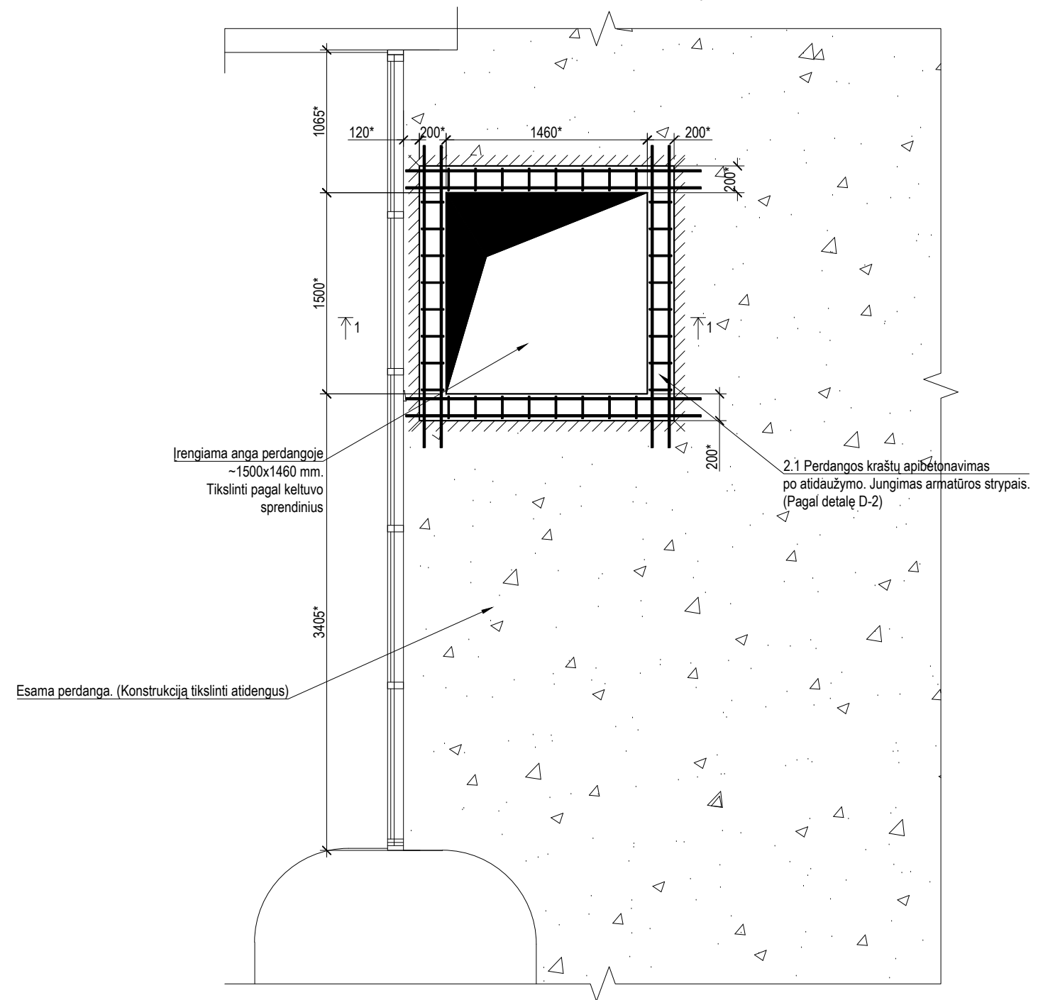
Pirmo aukšto perdangos planas naujai įrengiamo keltuvo zonoje M1:40
