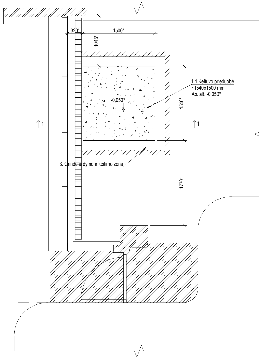
Keltuvo prieduobės planas M1:40
