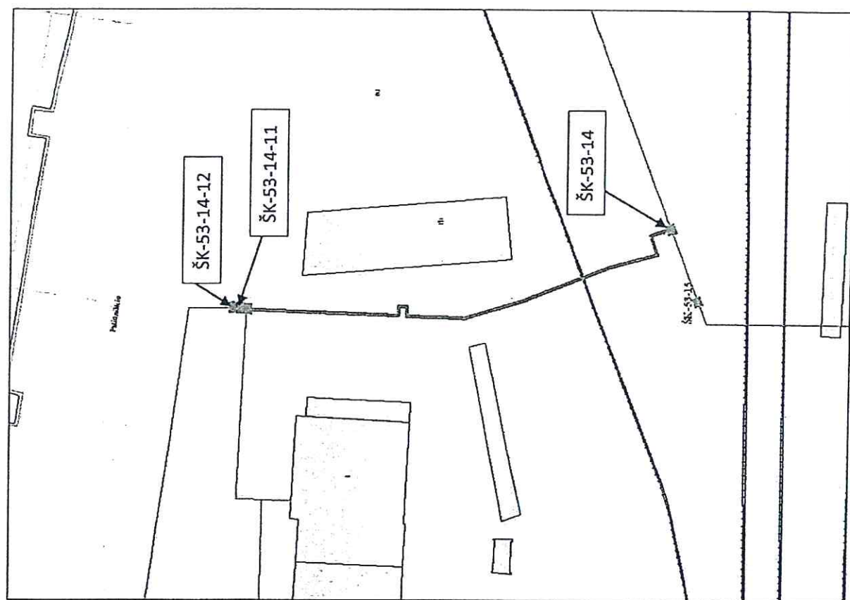
Šilumos tinklų nuo ŠK-53-14 iki ŠK-53-14-12 Panevėžyje situacijos schema
