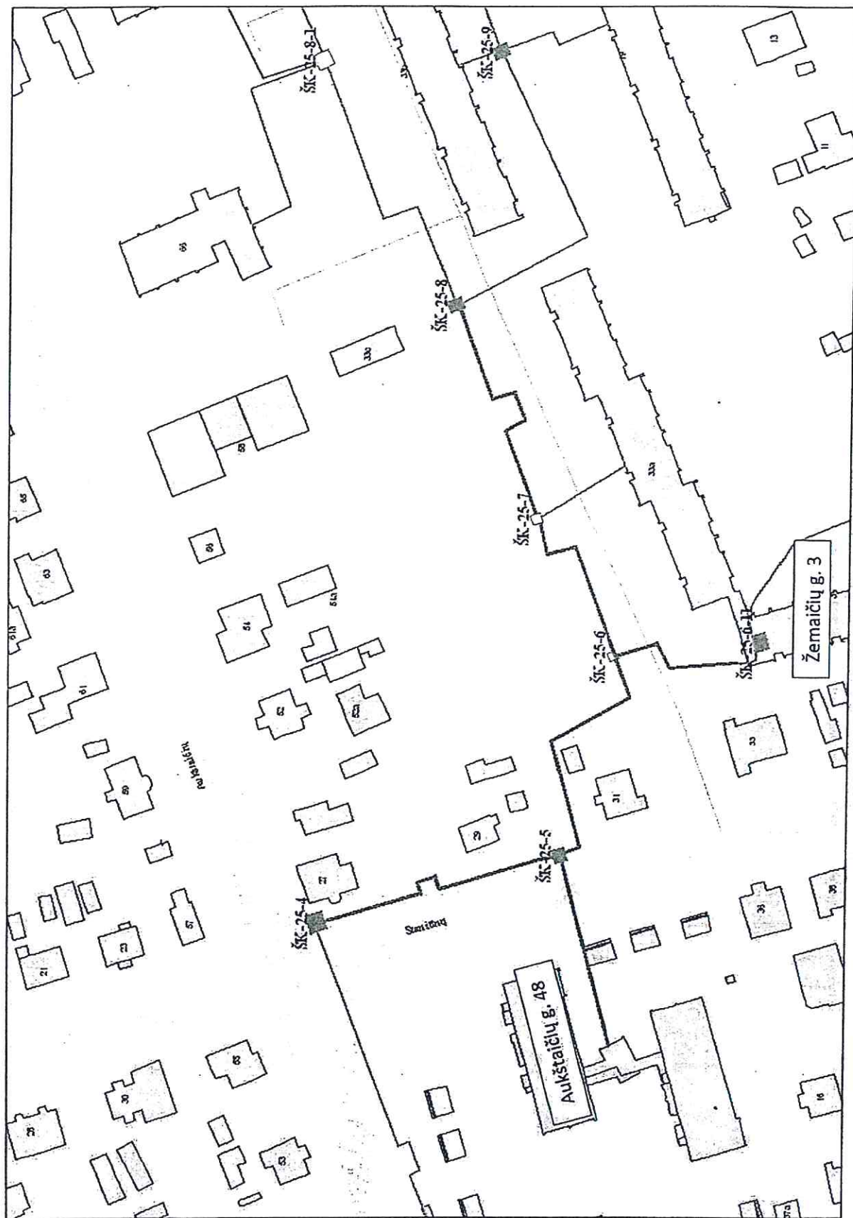
Šilumos tinklų nuo ŠK-25-4 iki ŠK-25-8 Panevėžyje situacijos schema
