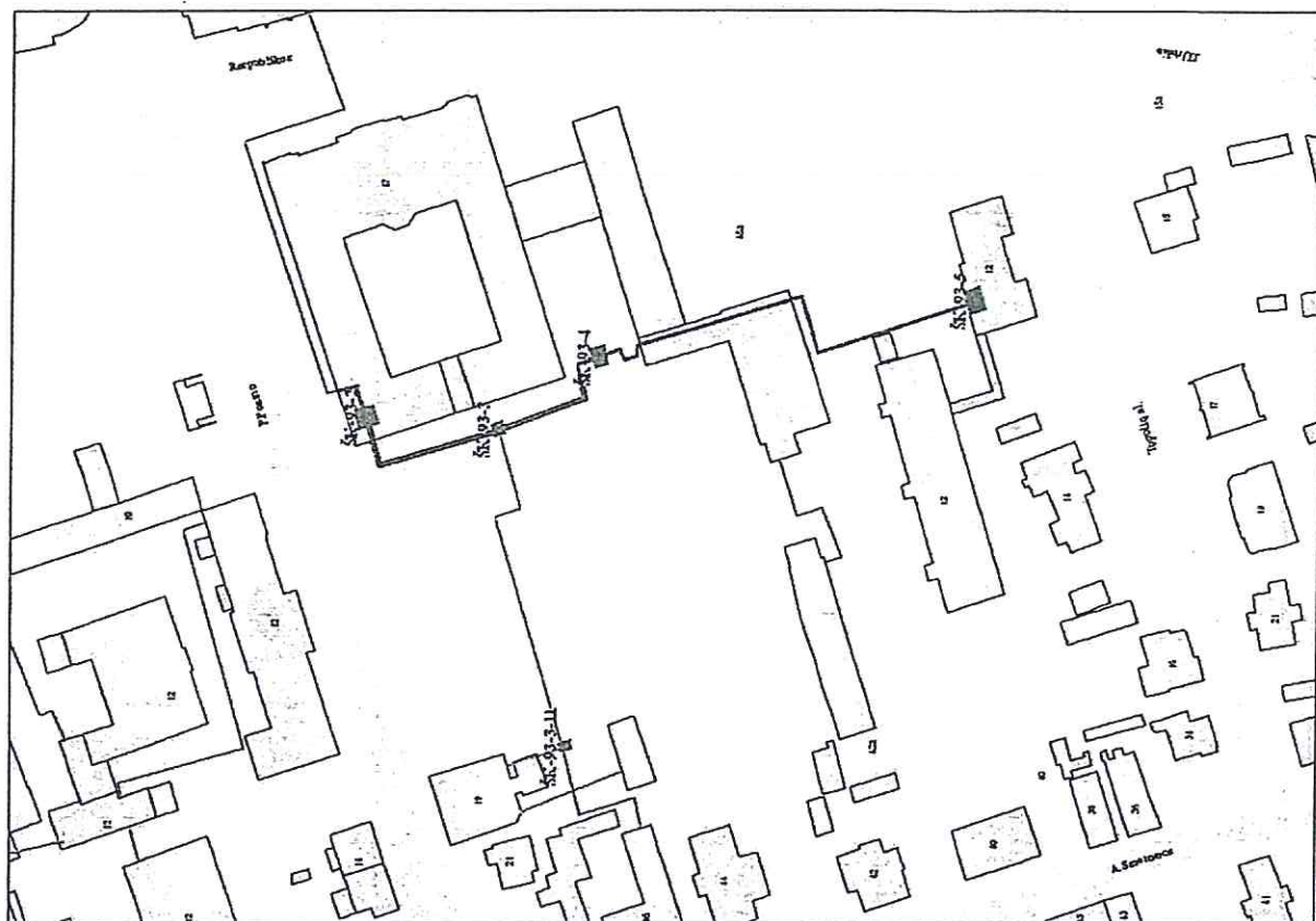
Šilumos tinklų nuo ŠK-93-2 iki ŠK-93-5 Panevėžyje situacijos schema
