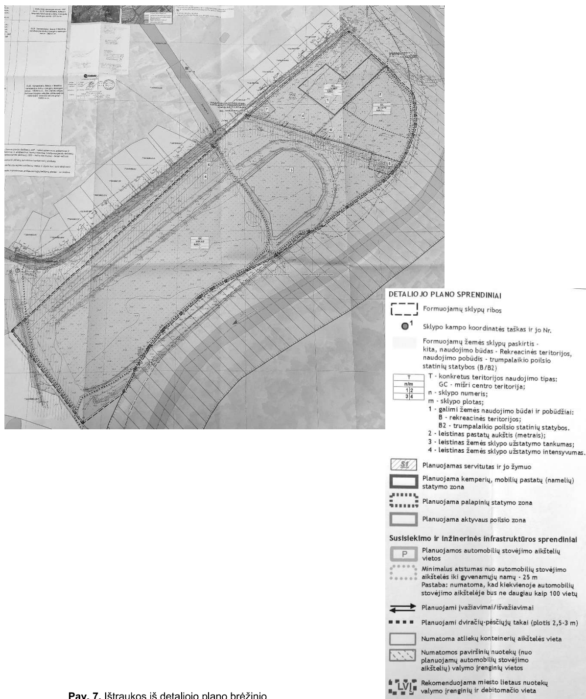
Pav. 7. Ištraukos iš detaliojo plano brėžinio
