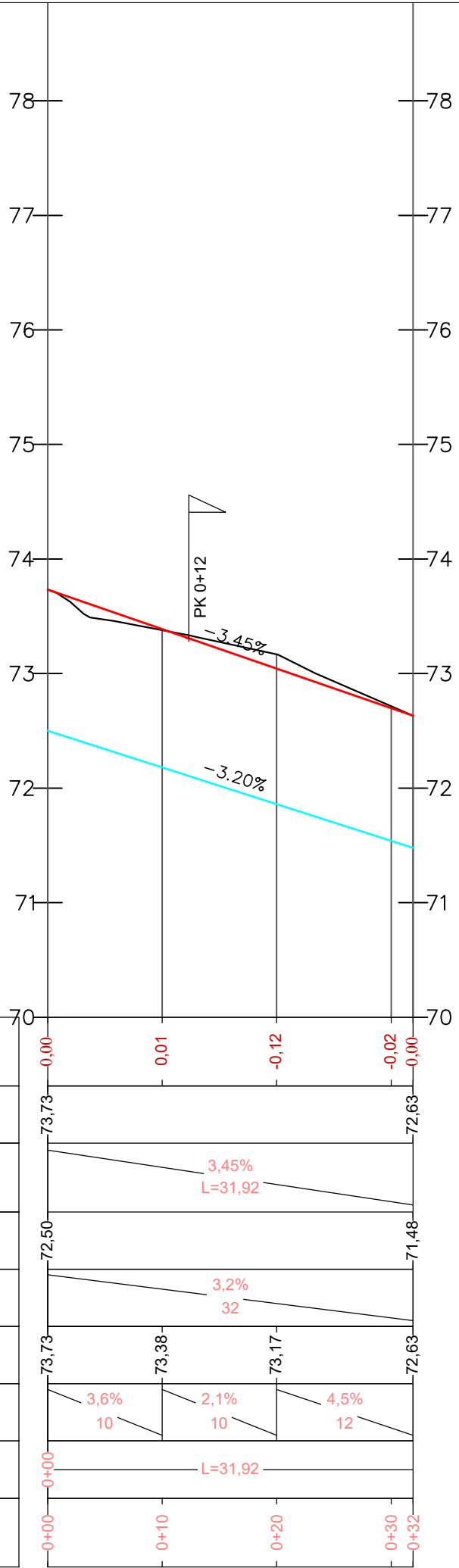
IŠILGINIS PROFILIS Mv 1:50 Mh 1:500
