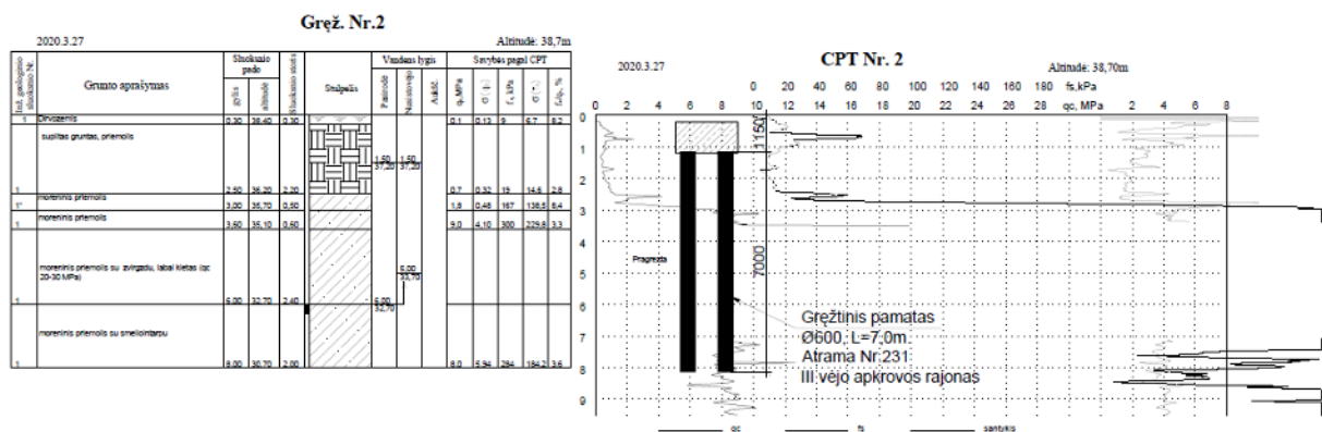
Pav. 1. Konstrukcinė pamatų schema ant geologinio pjūvio
