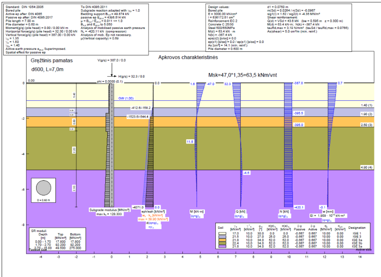
Pav. 5. Poliaus laikomosios galios tikrinimas nuo skersinės jėgos sudaromo momento
