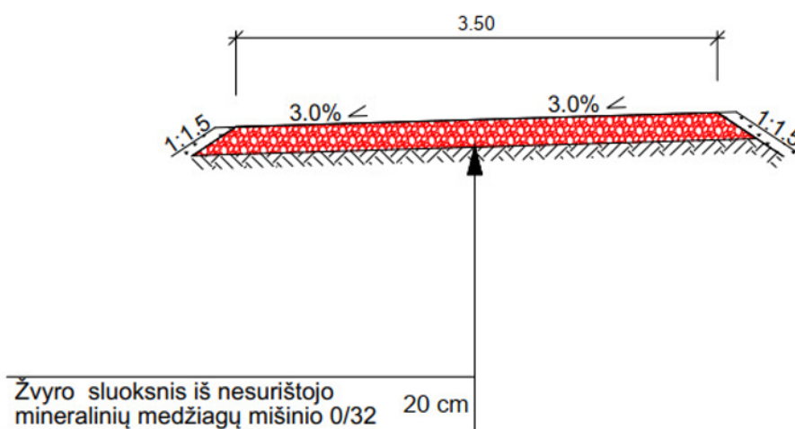
2 pav. Laikino privažiavimo dangos konstrukcija
