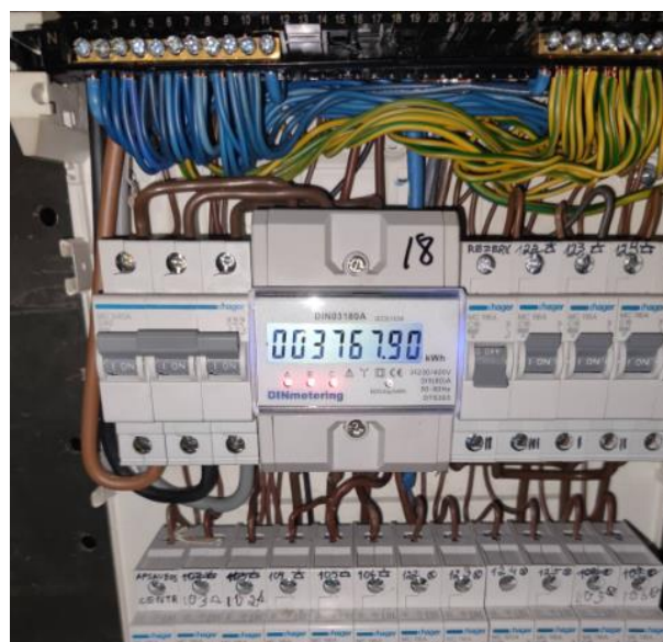
pav. 3 3F esamas elektros skaitiklis
