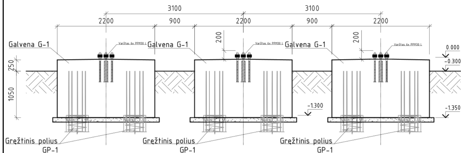
VAIZDAS 1-1 M1:50
