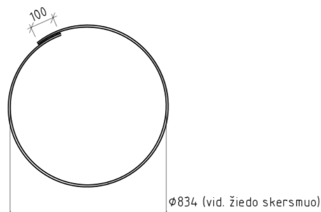
POZ. 3 M1:20
