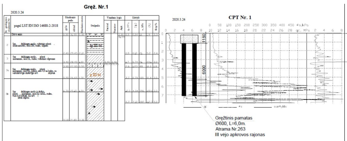
Pav. 1. Konstrukcinė pamatų schema ant geologinio pjūvio
