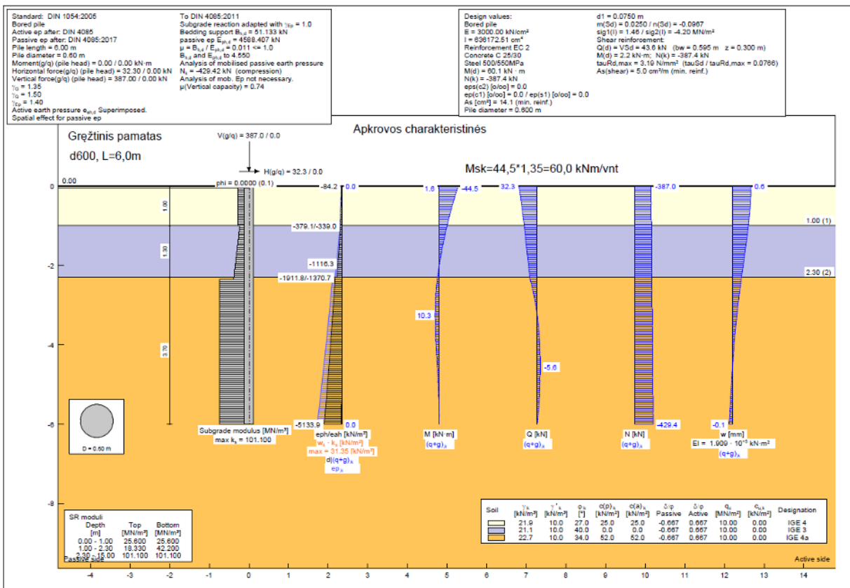
Pav. 5. Poliaus laikomosios galios tikrinimas nuo skersinės jėgos sudaromo momento
