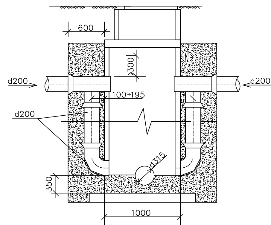
KAI ŠULINIO SKERSMUO D1000
