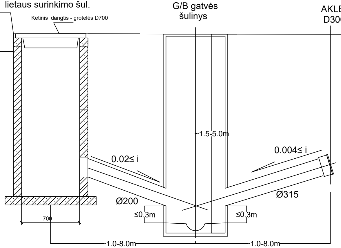
PJŪVIS C-C
