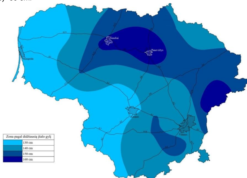
5 pav. Lietuvos teritorijos kartografinis zonavimas pagal didžiausią įšalo gylį
