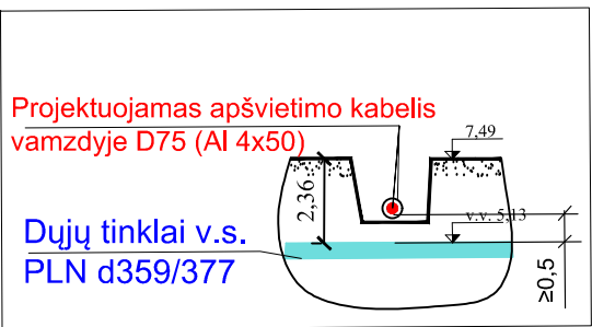
Pjūvis 14-14
