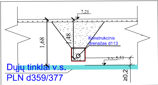
Pjūvis 17-17
