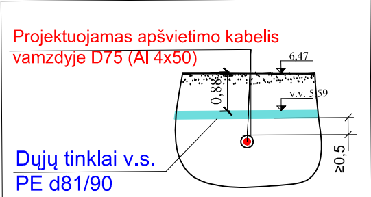
Pjūvis 8-8
