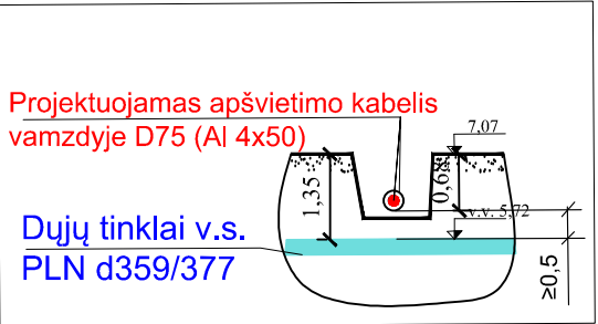
Pjūvis 18-18
