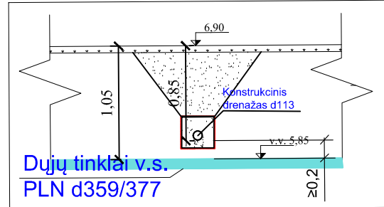
Pjūvis 19-19
