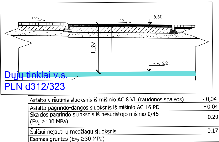
Pjūvis 10-10
