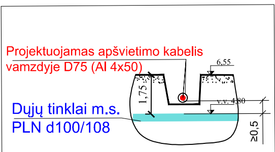
Pjūvis 13-13
