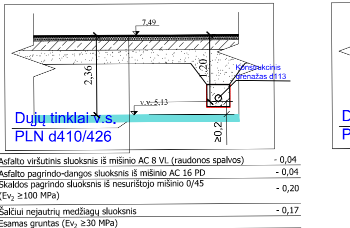
Pjūvis 19-19
