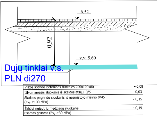
Pjūvis 7-7
