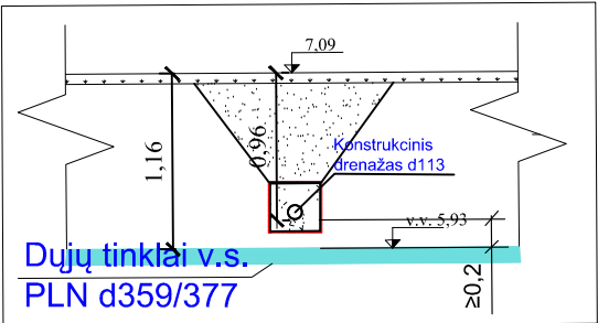
Pjūvis 20-20
