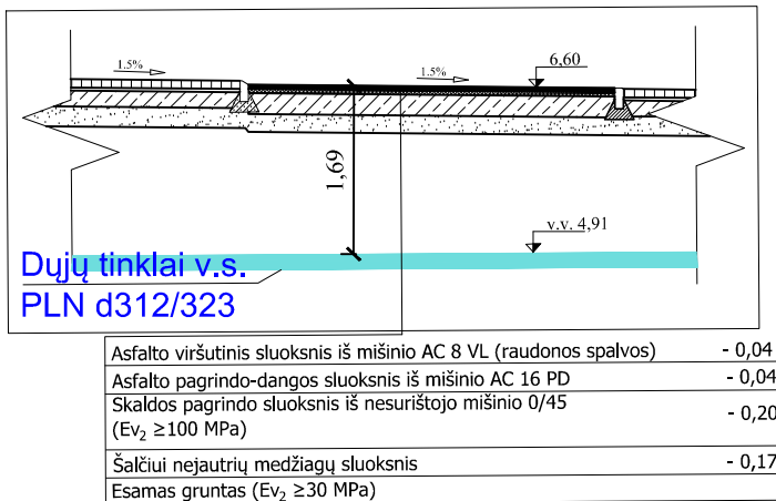
Pjūvis 15-15
