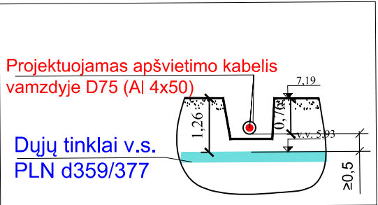
Pjūvis 21-21
