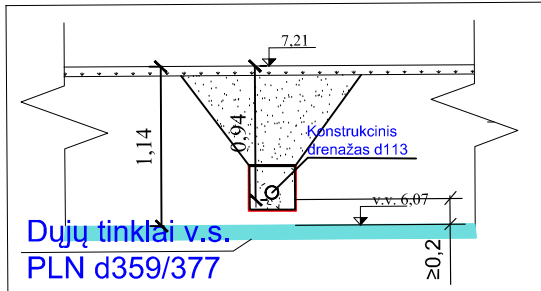
Pjūvis 16-16
